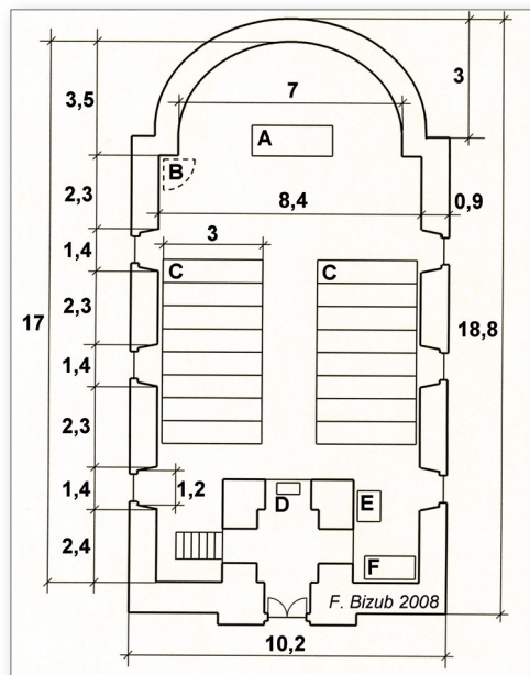
50. Pôdorys kaplnky
